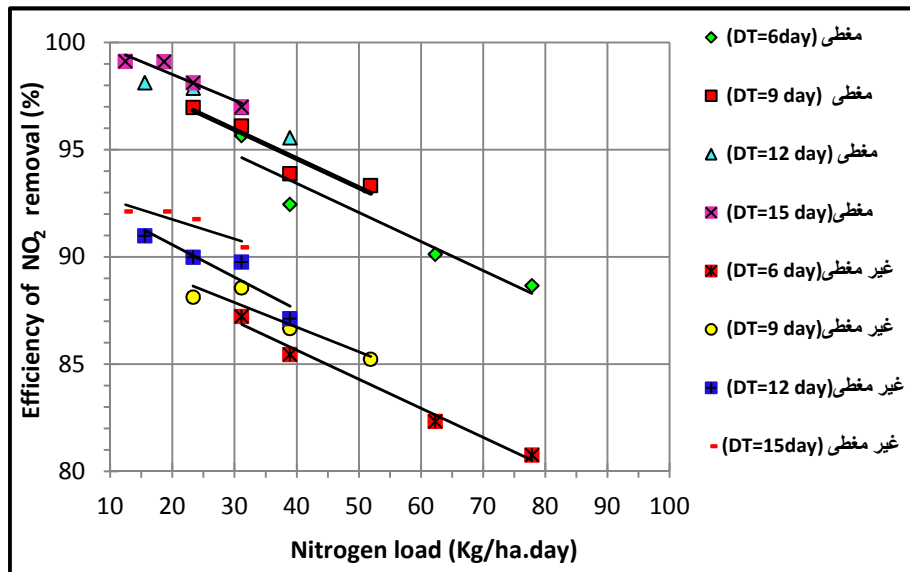
الشكل (2) : العلاقة بين الحمل النتروجيني المسلط على الوحدات الاختبارية وكفاءة إزالة النترات ( \text{NO}_2 )
