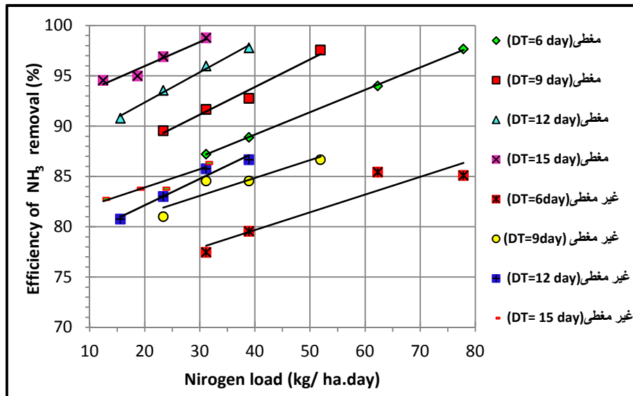
الشكل (1): العلاقة بين الحمل النتروجيني المسلط على الوحدات الاختبارية وكفاءة إزالة الأمونيا (NH 3 )
