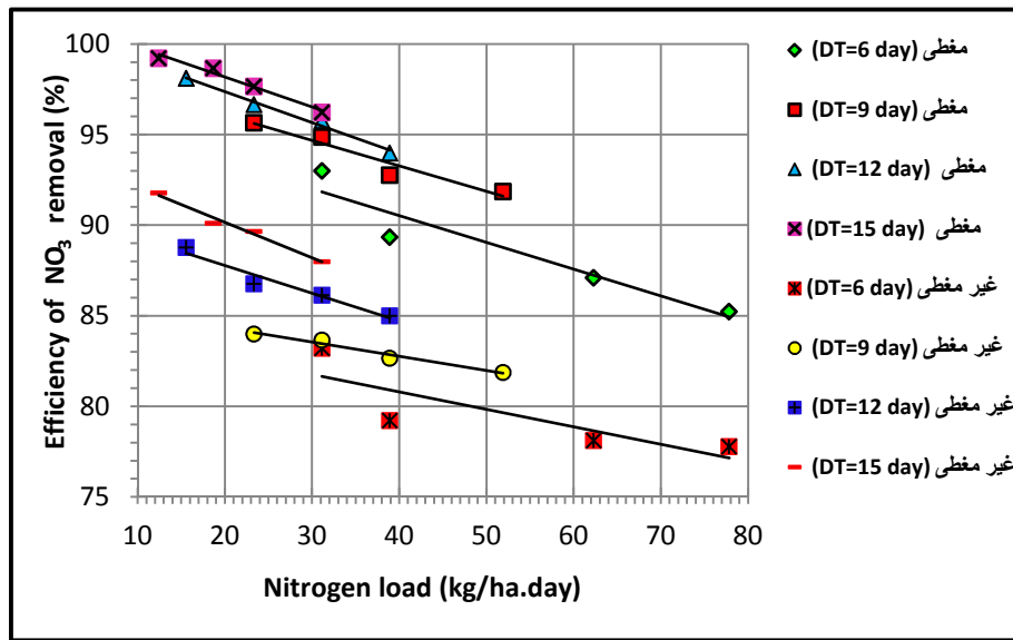
الشكل (3) : العلاقة بين الحمل النتروجيني المسلط على الوحدات الاختبارية وكفاءة إزالة النترات ( \text{NO}_3 )
