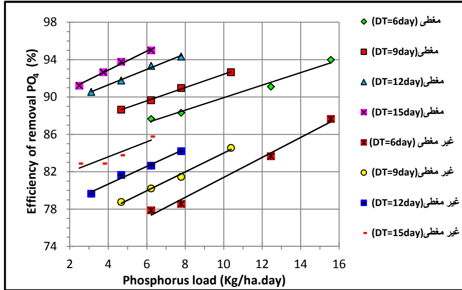
الشكل (4) : العلاقة بين أحمال الفسفور المسلطة على الوحدات الاختبارية وكفاءة إزالة الفوسفات ( PO_4 )
