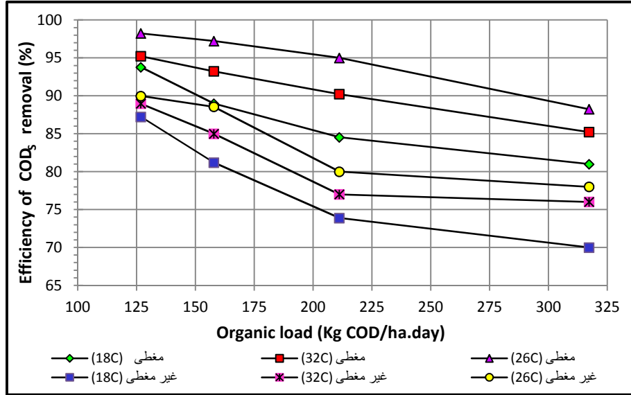
الشكل (5) : العلاقة بين الحمل العضوي المسلط على الوحدات الاختبارية وكفاءة إزالة المواد العضوية المذابة (COD 5 )
