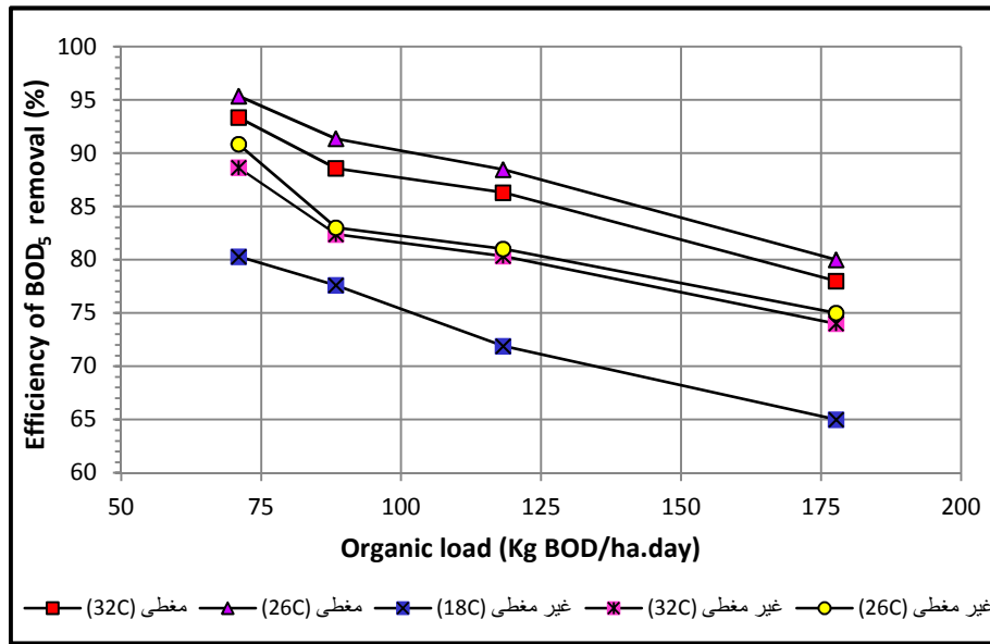
الشكل (6) : العلاقة بين الحمل العضوي المسلط على الوحدات الاختبارية وكفاءة إزالته المواد العضوية (BOD 5 )
